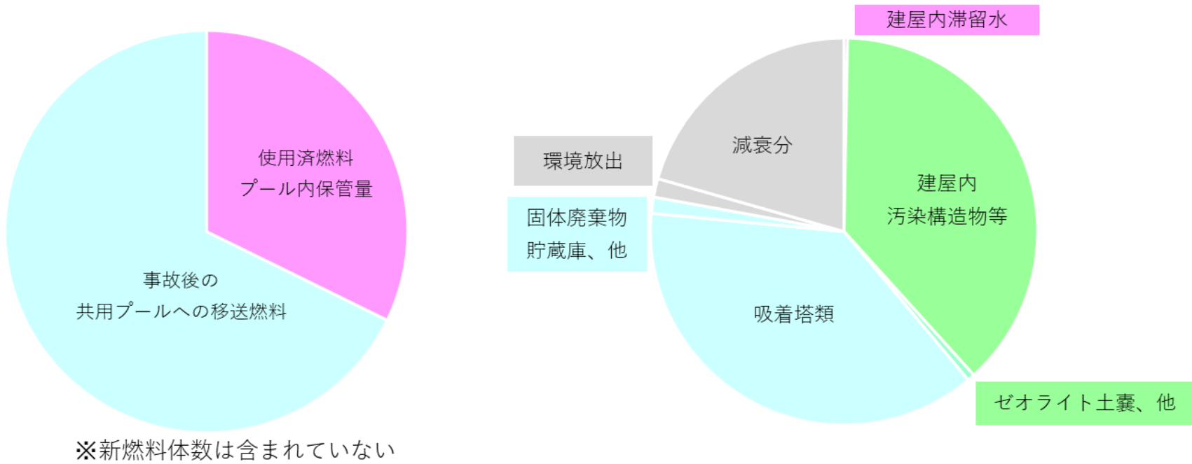
(c) 事故時に放出されたCs-137の放射能 (1号機～3号機)
